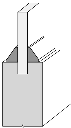
Optional bevel bead
